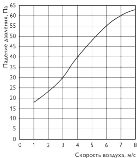
КПО 300x150, КПО 400x200 КПО 500x300, КПО 600x300
