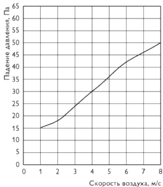
КПО 600x350, КПО 700x400 КПО 800x500, КПО 1000x500
