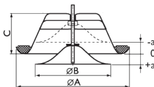
Размеры, мм
