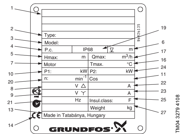
Рис. 3 SL1 и SLV кроме SL1.50.65.09/11/15 и SLV.65.65.09/11/15
