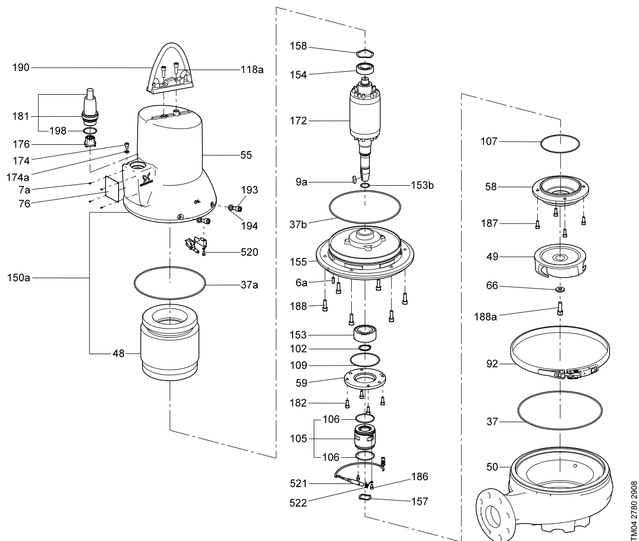
Рис. 21 Деталировки, SLV.65.65.22/30/40, SLV.65.80.xx, SLV.80.80.xx, SLV.80.100.xx, SLV.100.100.xx с датчиком
