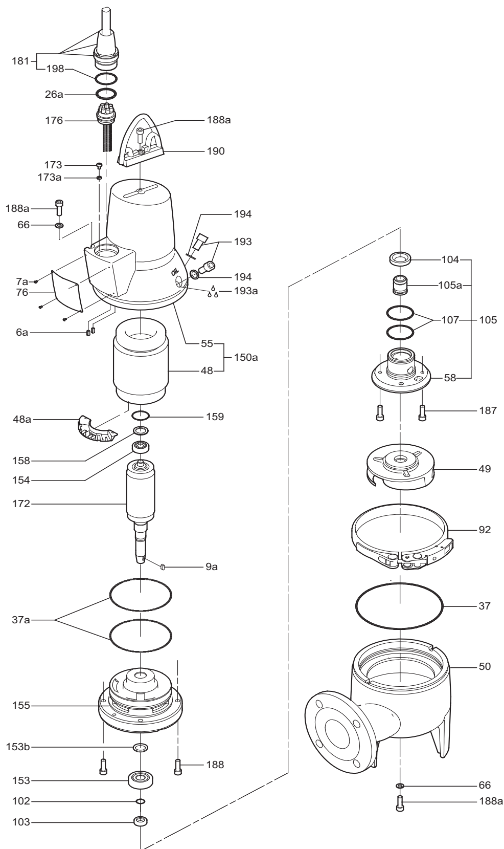
Рис. 17 Деталировки, SLV.65.65.09/11/15
