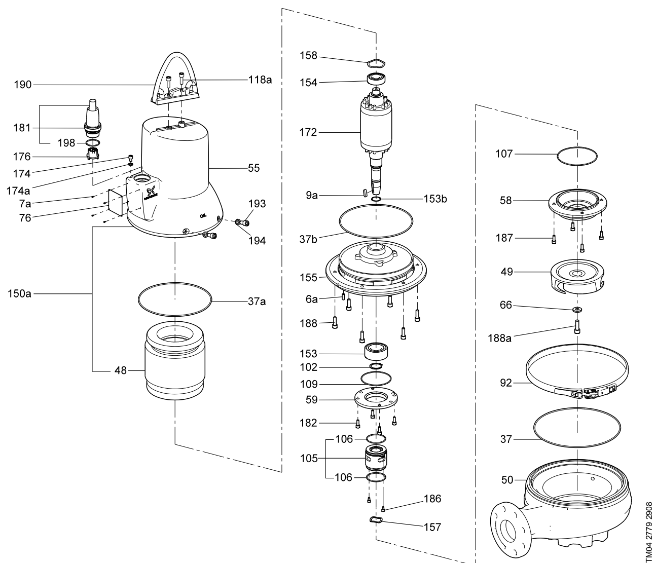
Рис. 19 Чертёж в разрезе, SLV.65.65.22/30/40, SLV.65.80.xx, SLV.80.80.xx, SLV.80.100.xx, SLV.100.100.xx без датчика
