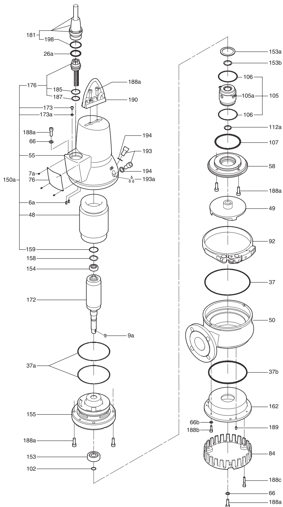
Рис. 7 Деталировки, DP10.65.26
