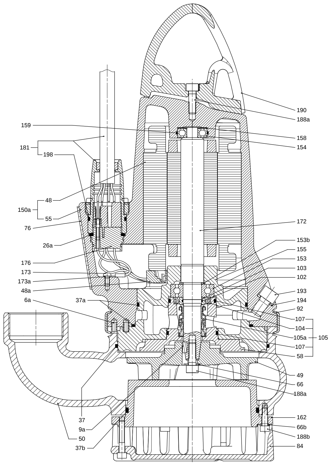
Рис. 4 Чертёж в разрезе, DP10.50.09/15
