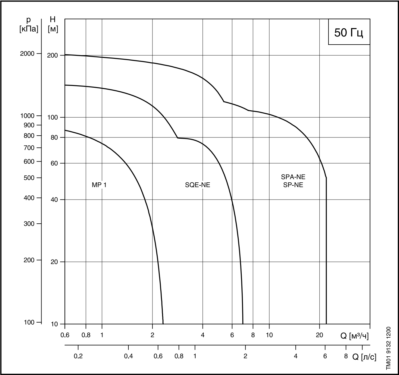
Диаграммы рабочих характеристик насосов
