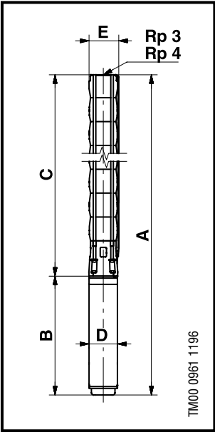
Насосы моделей от SP 46–26 до SP 46–33 устанавливают в кожухе с присоединением R4.
