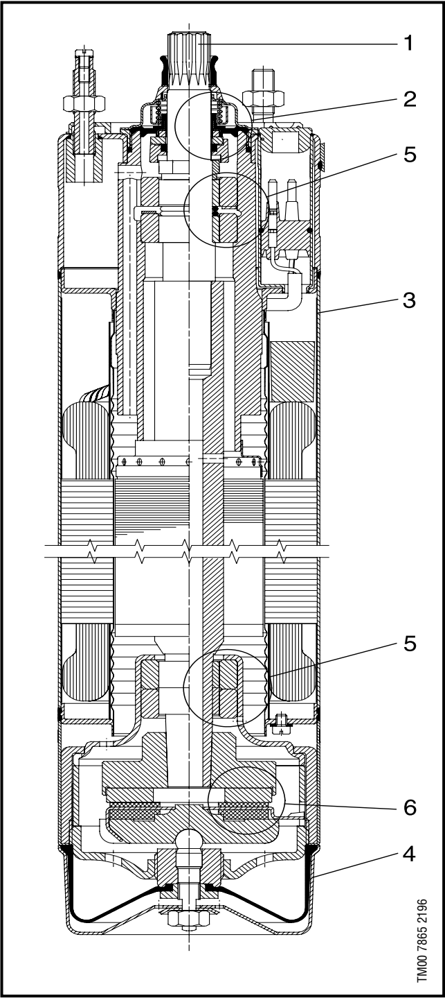
Продольное сечение: MS 4000
