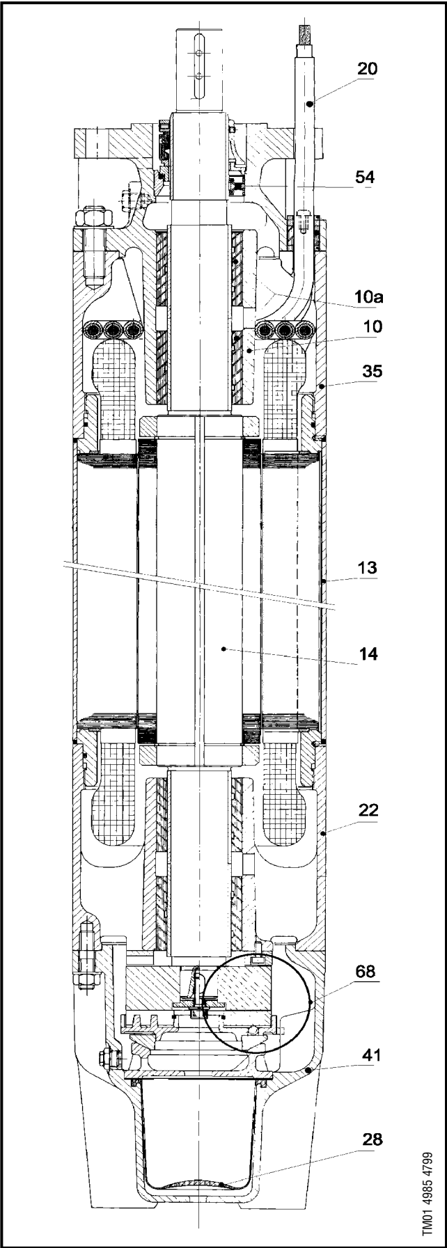
Продольное сечение: MMS 10000
