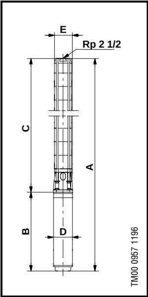
Насосы моделей от SP 17– 43 по SP 17– 48 устанавливают в кожухе с присоединением R3.
