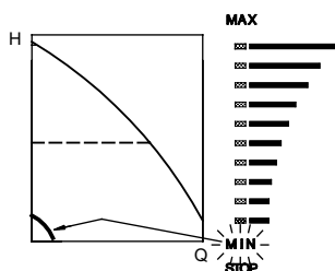
Рис. 19 Мин. характеристика
