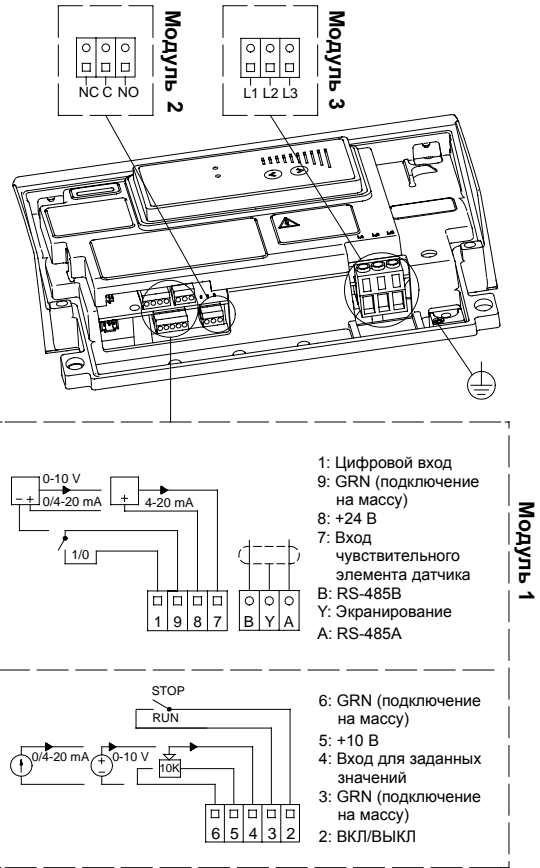
Рис. 4 Схема соединений – TPE
