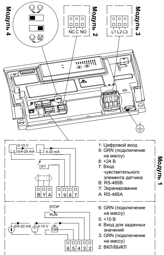
Рис. 5 Схема соединений – TPED
